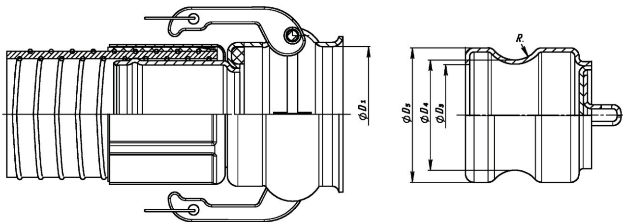
Головка присоединительная
