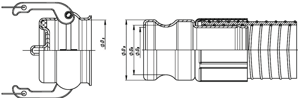
Рисунок 14 – Присоединительные размеры адаптеров:
