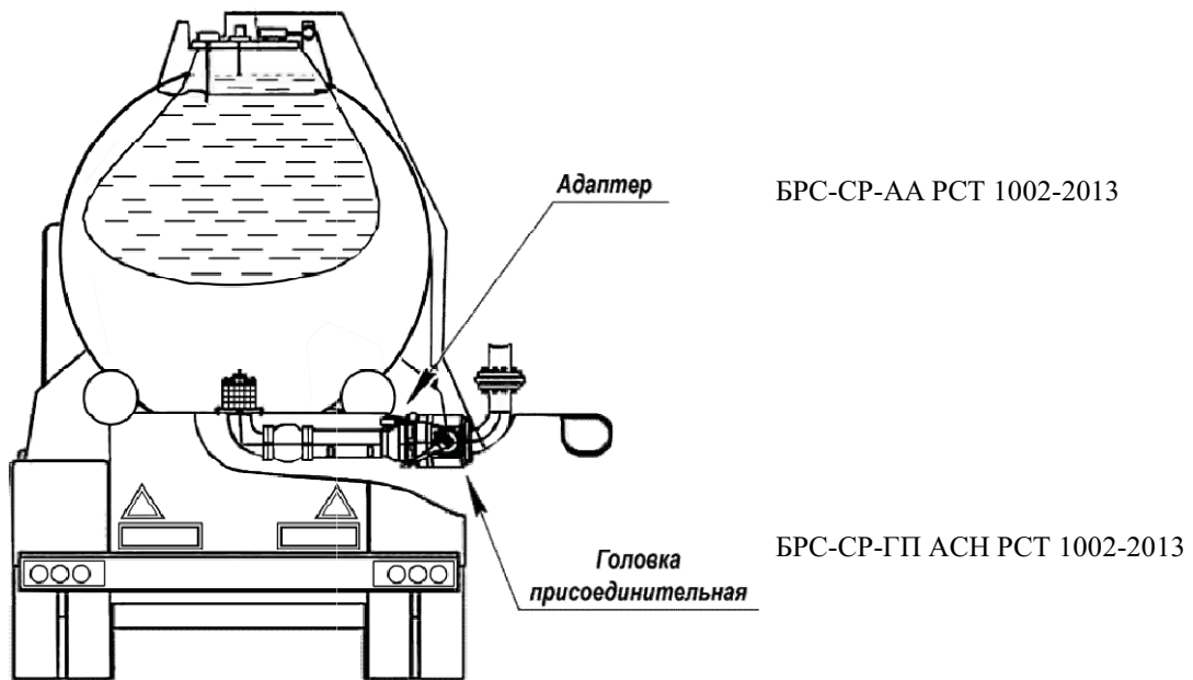
Рисунок 16 – Пример применения сухого разъёма
