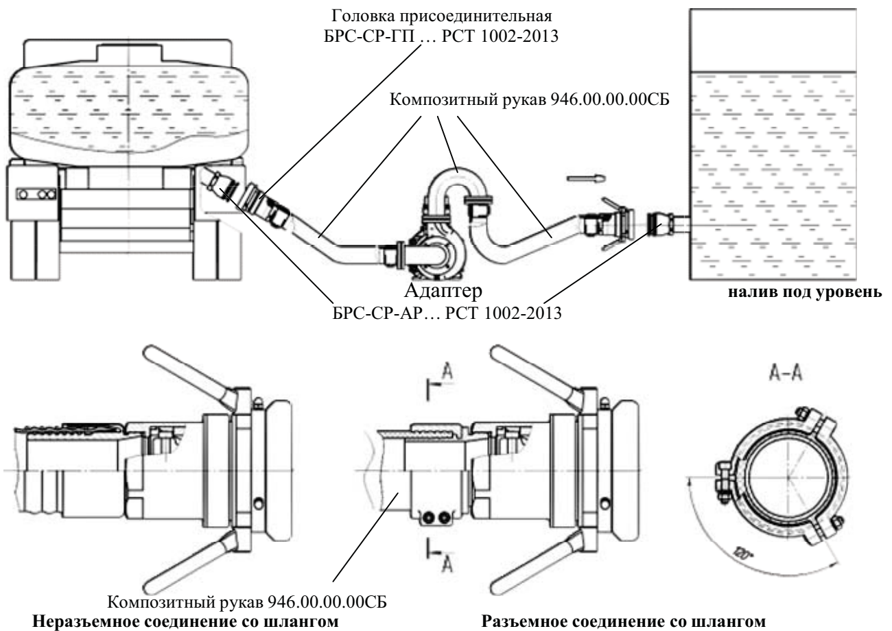
Рисунок 17 – Пример применения БРС-СР «ПРОМПРИБОР-ИТ»
