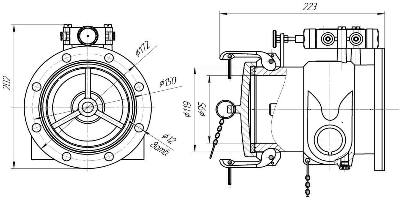
Рисунок 7 – Клапан паровозврата 1021.00.00.00. БРС типа БРС-ПВС
