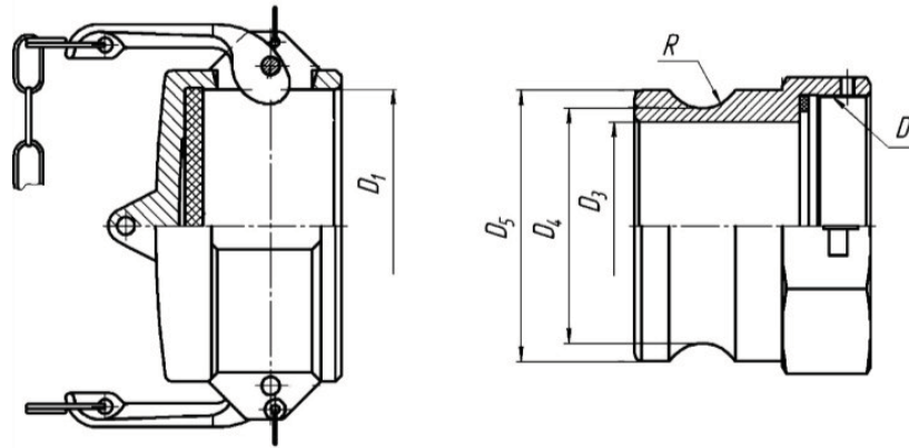
Заглушка к адаптеру
