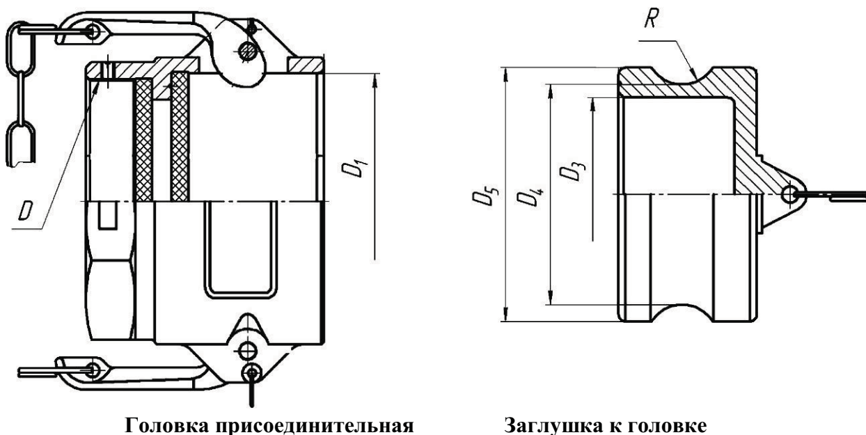
Рисунок 11 – Пристыковочные и присоединительные размеры головок присоединительных с кулачковой муфтой:
